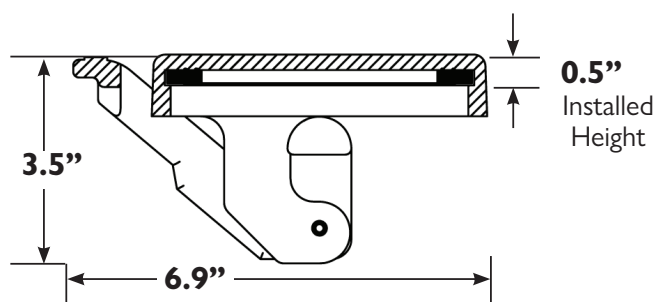
A0097-004LP Low Profile Fill Cap
